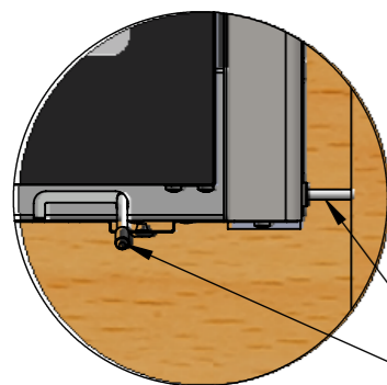
DETTAGLIO B SCALA 1 : 4
