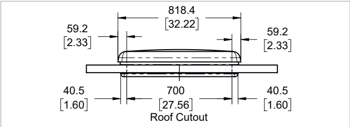
SKYMAXX LX PLUS (LED) - LED-EINHEIT 12V DC
